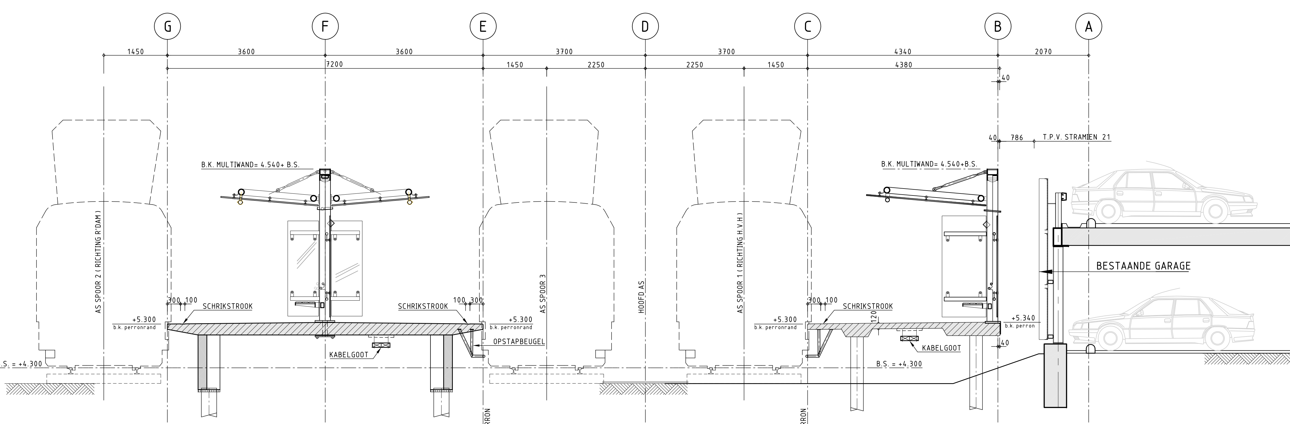
DOORSNEDE B-B SCHAAL 1:50
