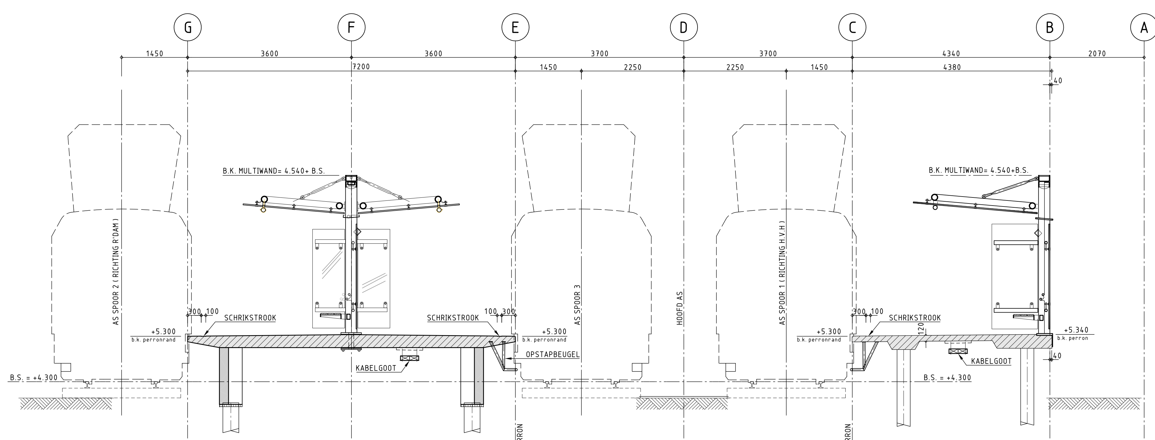
DOORSNEDE A-A SCHAAL 1:50
